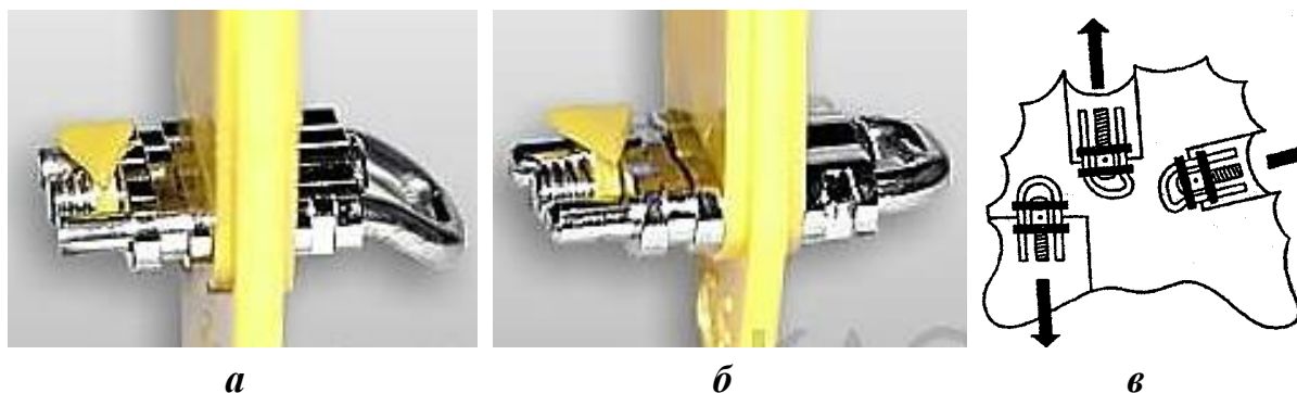
Рис. 84. Скелетированный винт с П-образной направляющей: а — изогнутый; б — прямой; в — схематическое изображение положения в аппарате
