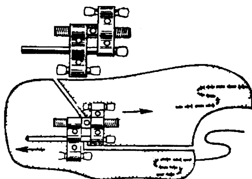
Рис. 96. Реципрокный винт Веллера
