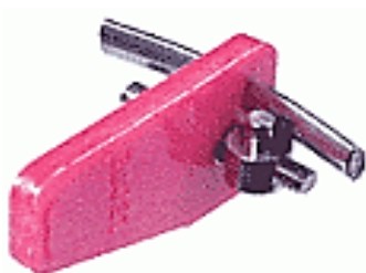
Рис. 90. Бюгельный винт Филиппа: а — внешний вид; б — схематическое изображение положения в аппарате в аппарате
